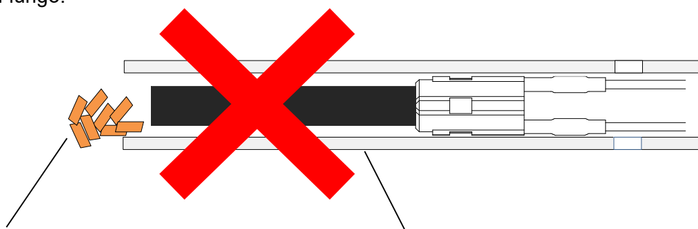
Elemento riscaldante troppo vicino a residui solidi di combustibile = rischio di contatto
