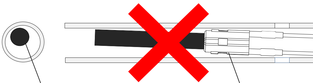
Elemento riscaldante inclinato a causa di difetti della fissazione
